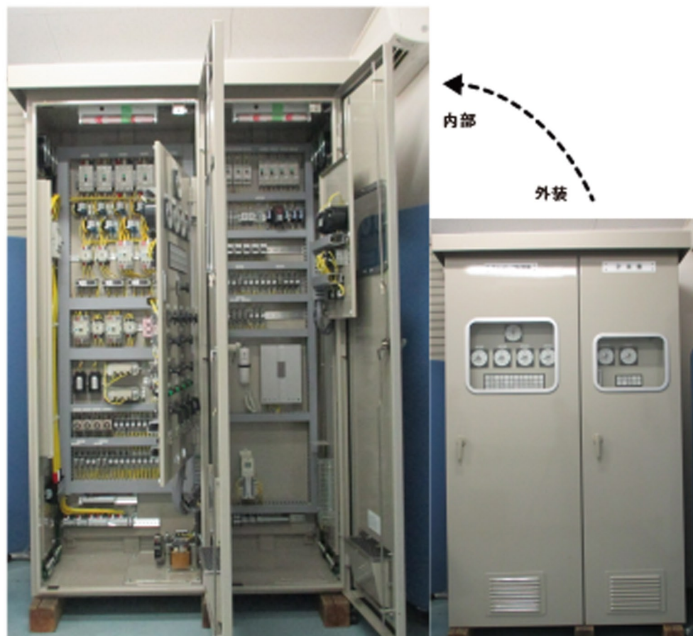
▲左側:汚水ポンプ制御盤、右側:計装盤
